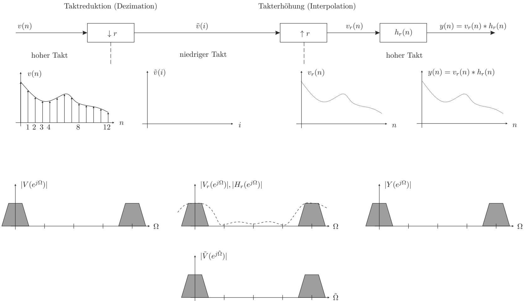
Abbildung 1: Zusatz 3 (Abtastratenumsetzung)
