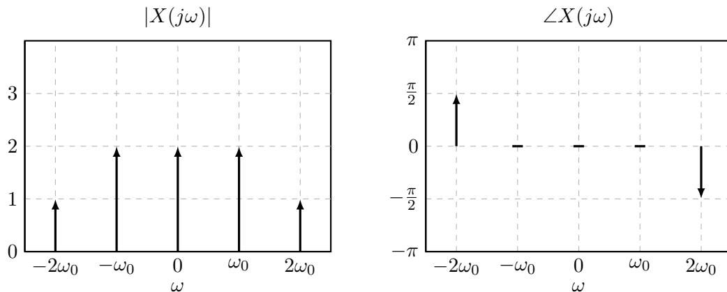
Abbildung 1: Spektrum X(j\omega) des Signals x(t) .
